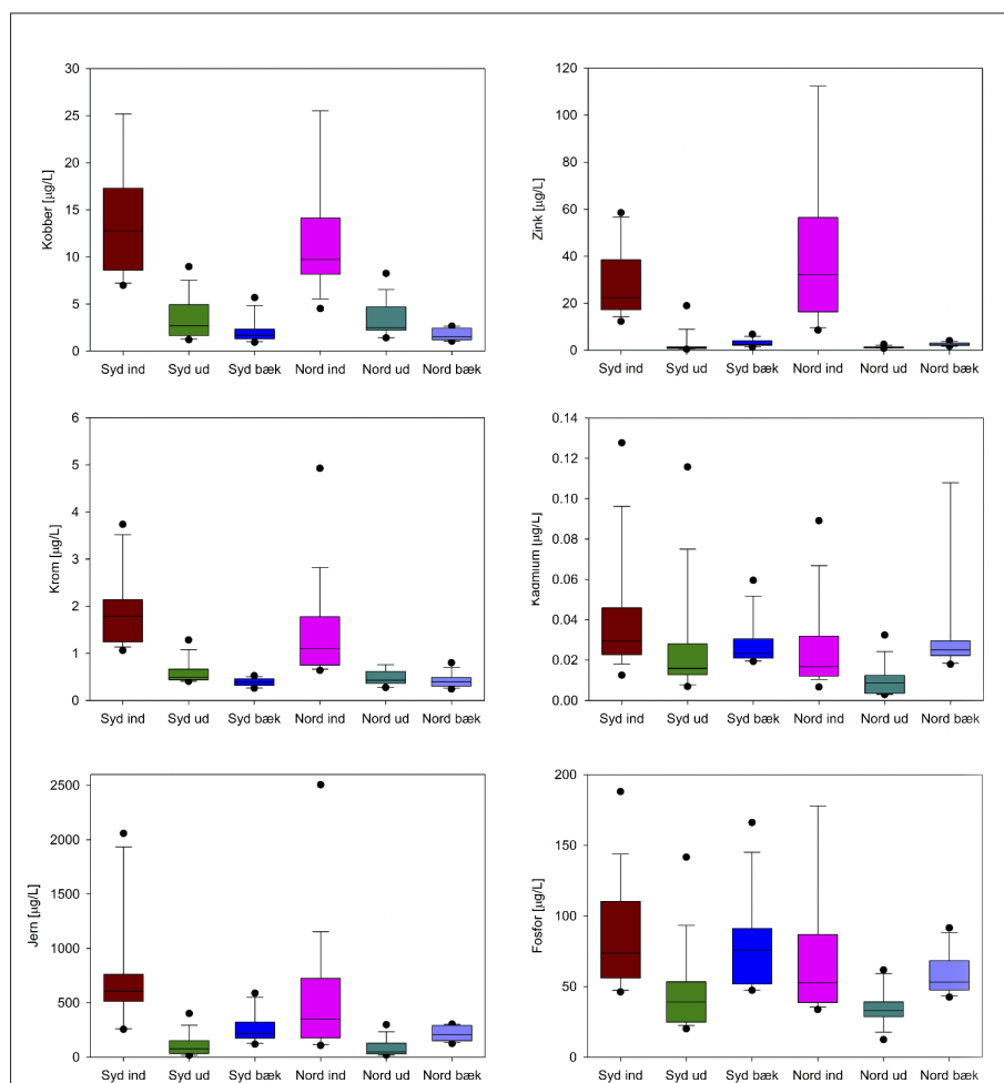
Figur 4. Fjernelse af stof i filteret sammenholdt med målte koncentrationer i Korskær Bæk. Data fra 2017.
