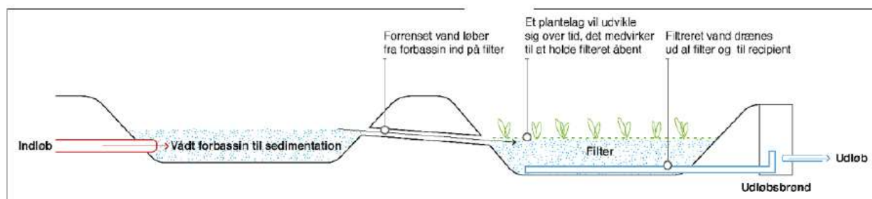
Figur 10 vådbassin med adsorptionsfilter i forlængelse
