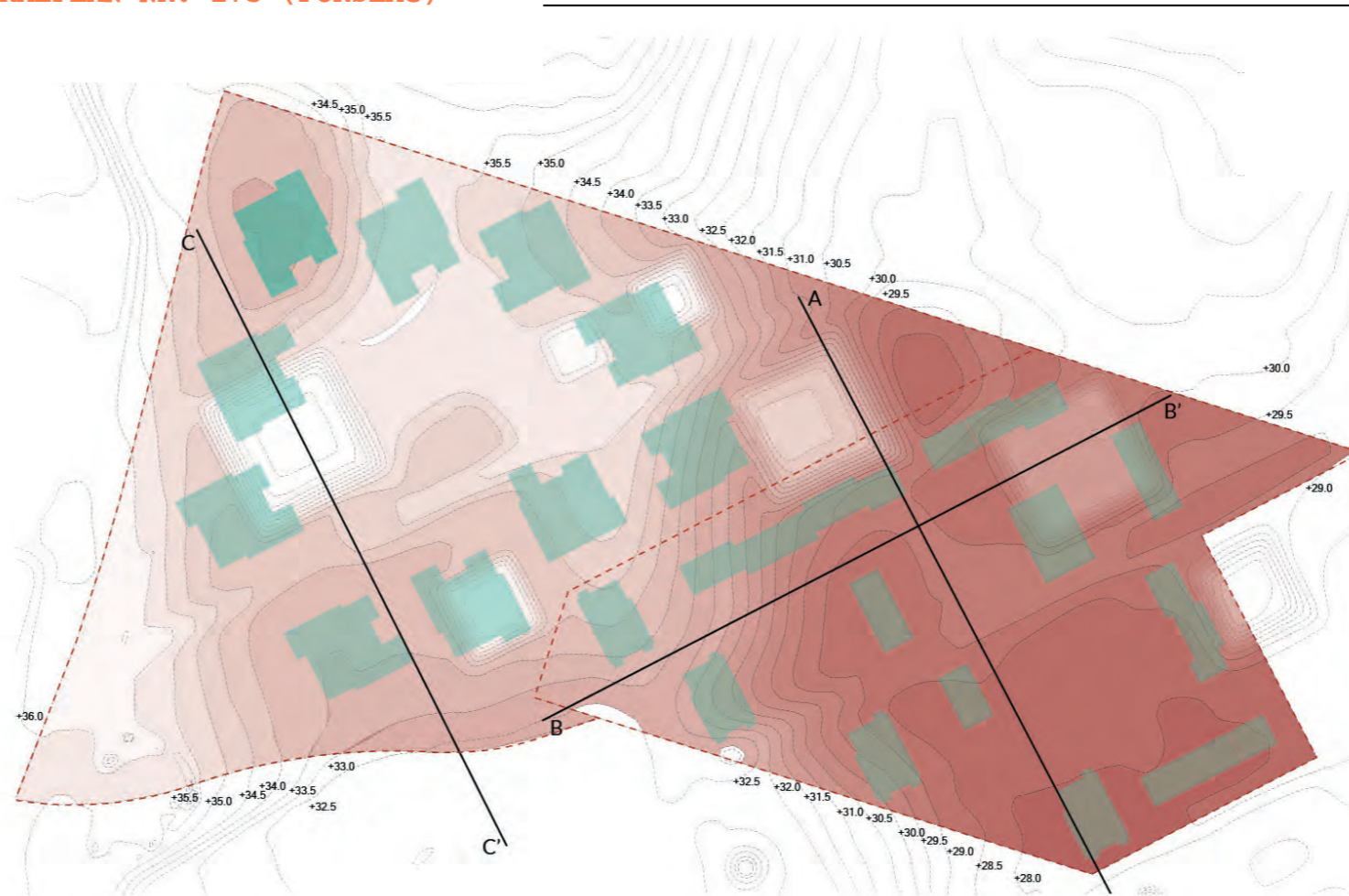
Eksisterende terræn
