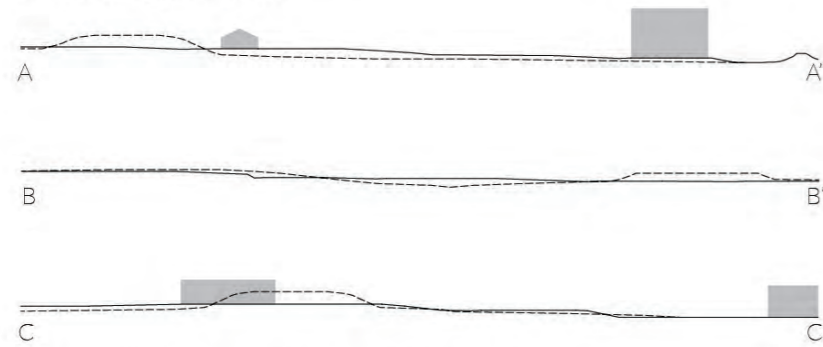
Terrænsnit - stiple linje er eksisterende terræn
