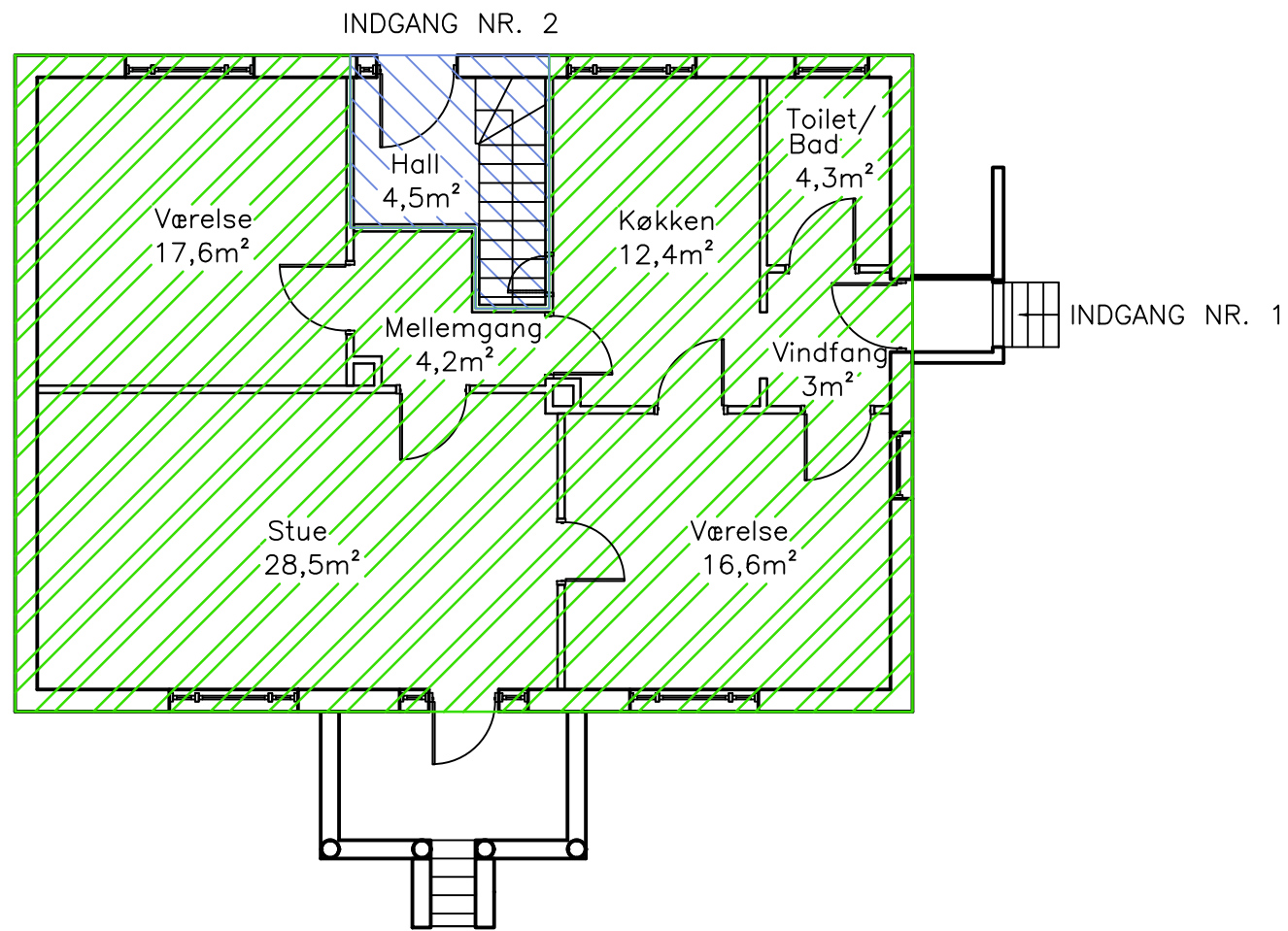
Stueplan, Hovedhus
