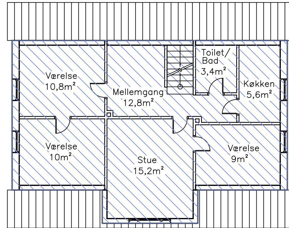
1.Salsplan, Hovedhus
