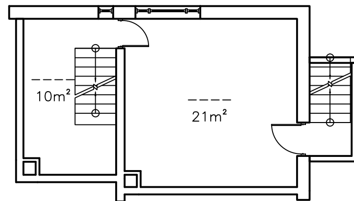
Kælderplan, Hovedhus
