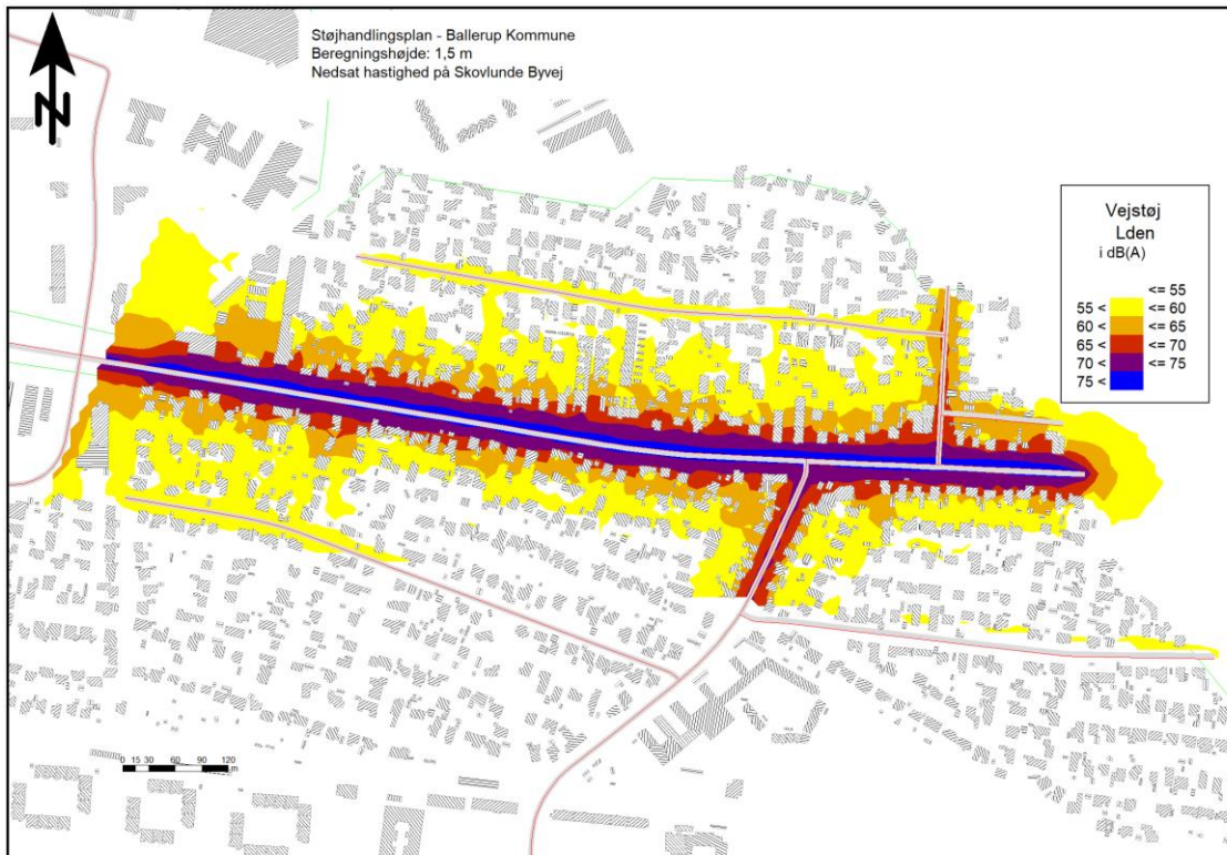
Figur 13: Støjudbredelse i 1,5 m højde langs Ballerup Boulevard med hastighedsreduktion
