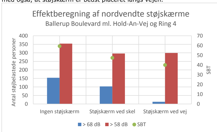
Figur 7: Effekt af nordvendte støjskærme på Ballerup Boulevard
