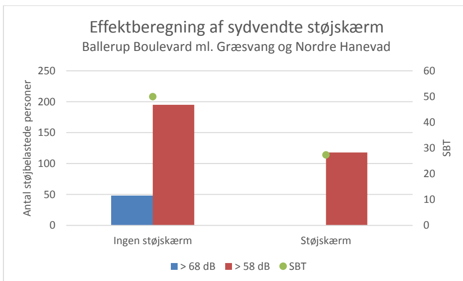
Figur 15: Effekt af sydvendt støjskærm på Ballerup Boulevard
