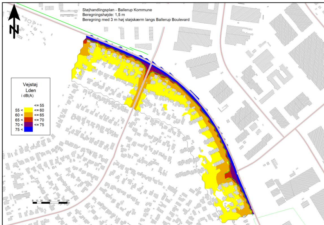
Figur 17: Støjudbredelse i 1,5 m højde langs Skovlunde Byvej med sydvendt støjskærm
