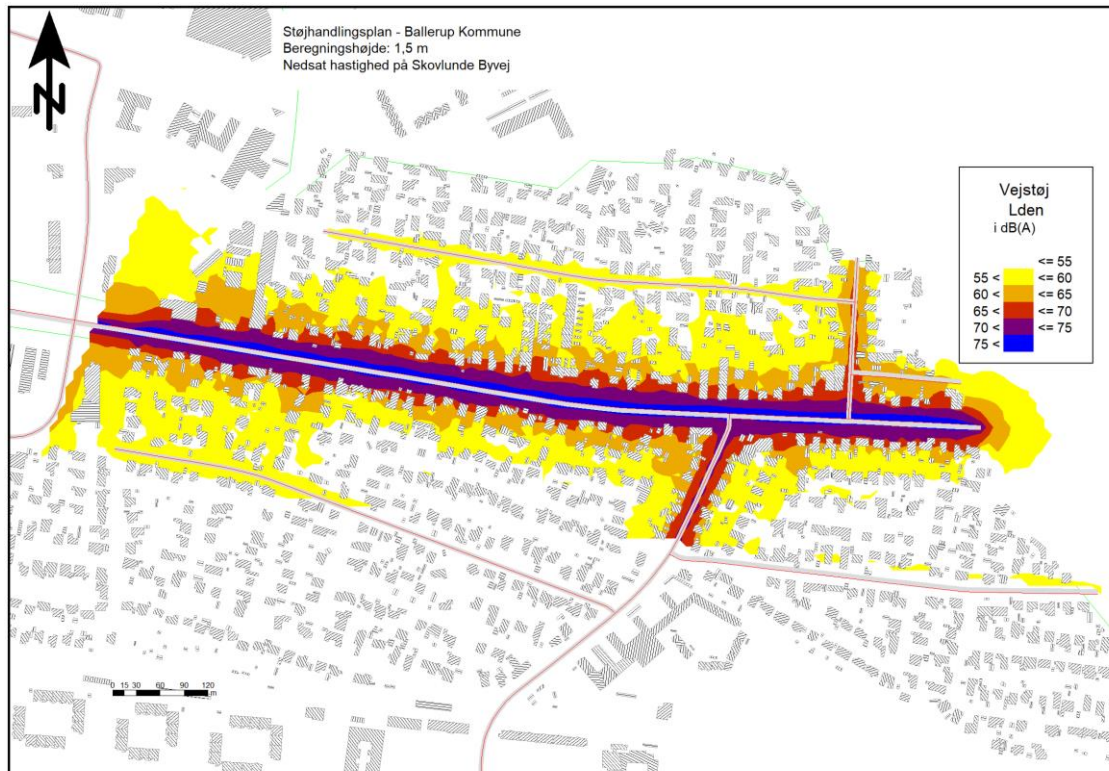
Figur 13: Støjuddbredelse i 1,5 m højde langs Ballerup Boulevard med hastighedsreduktion
