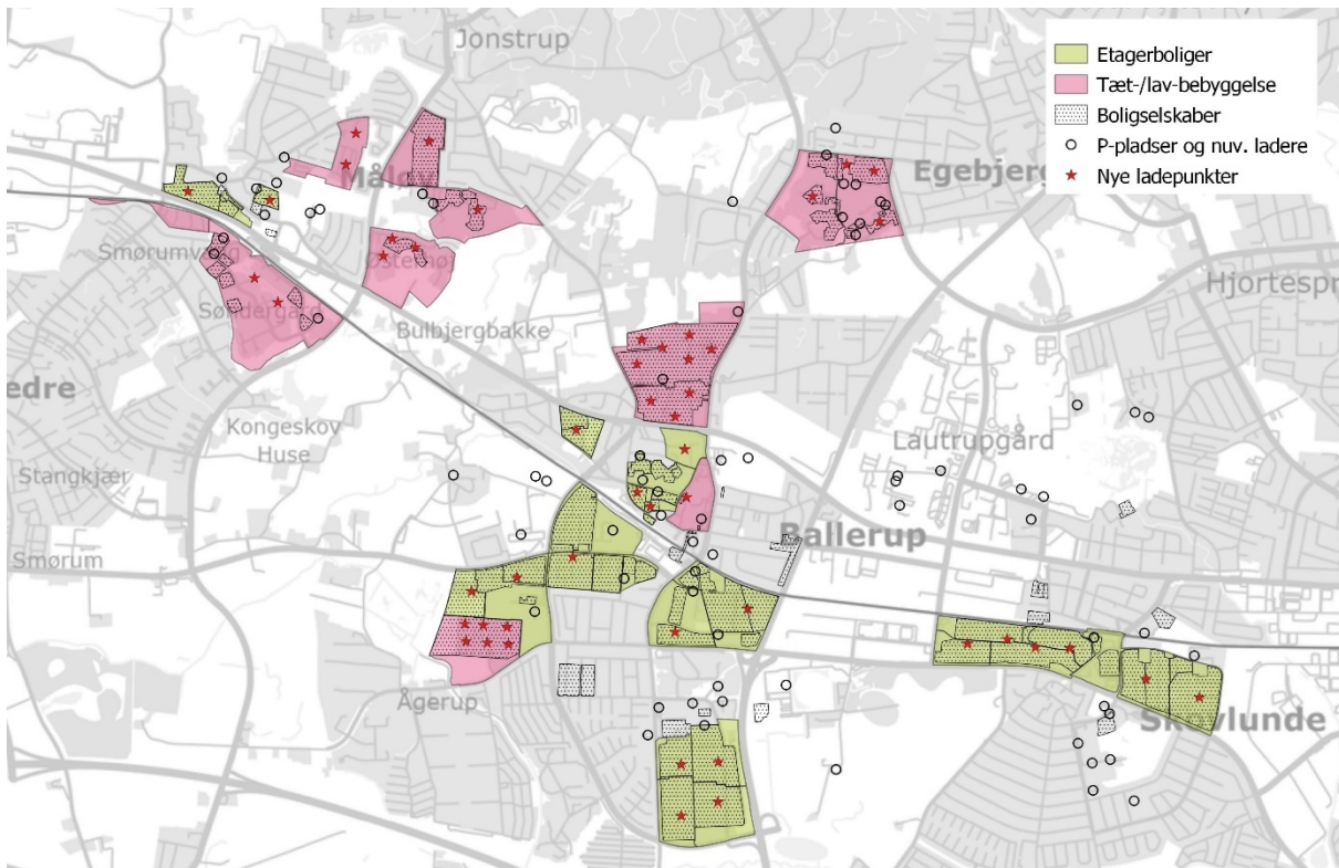
Figur 2: Optimal placering af 50 nye ladestationer.
