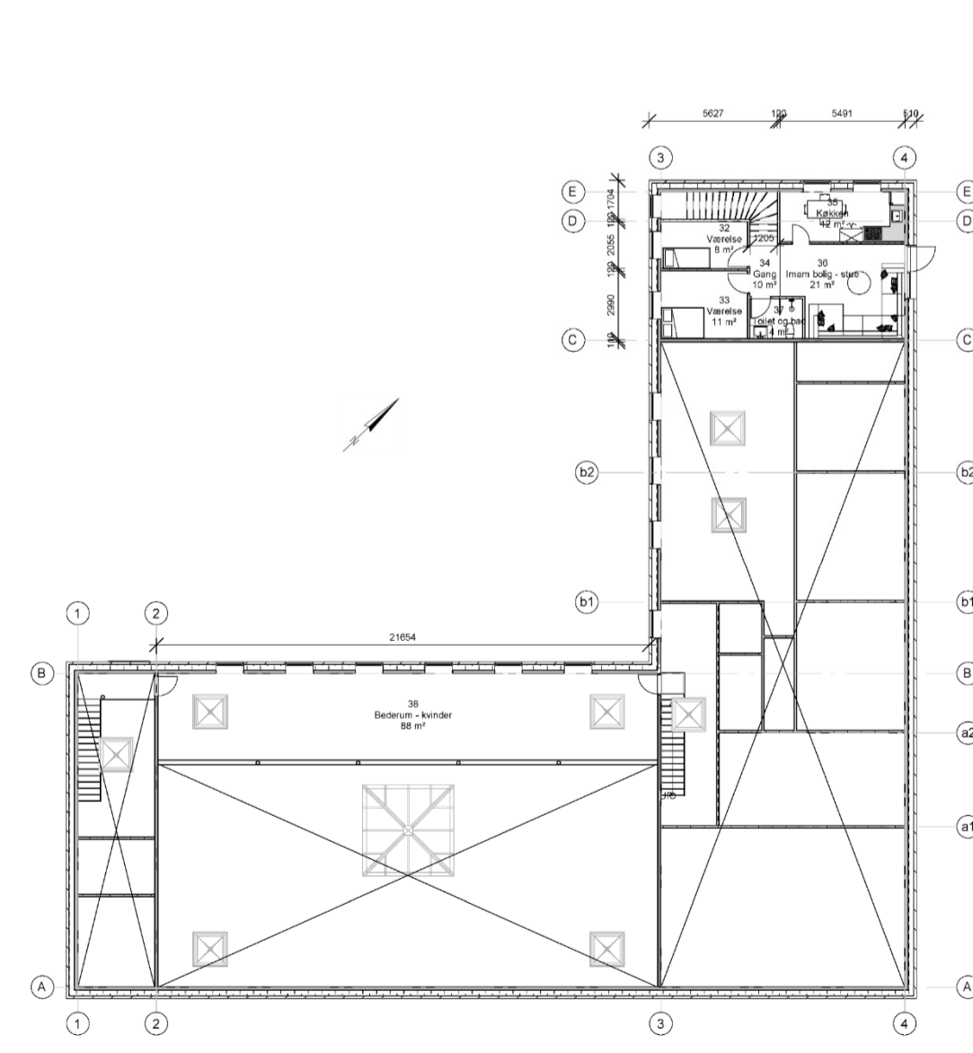
1. sal-plan
