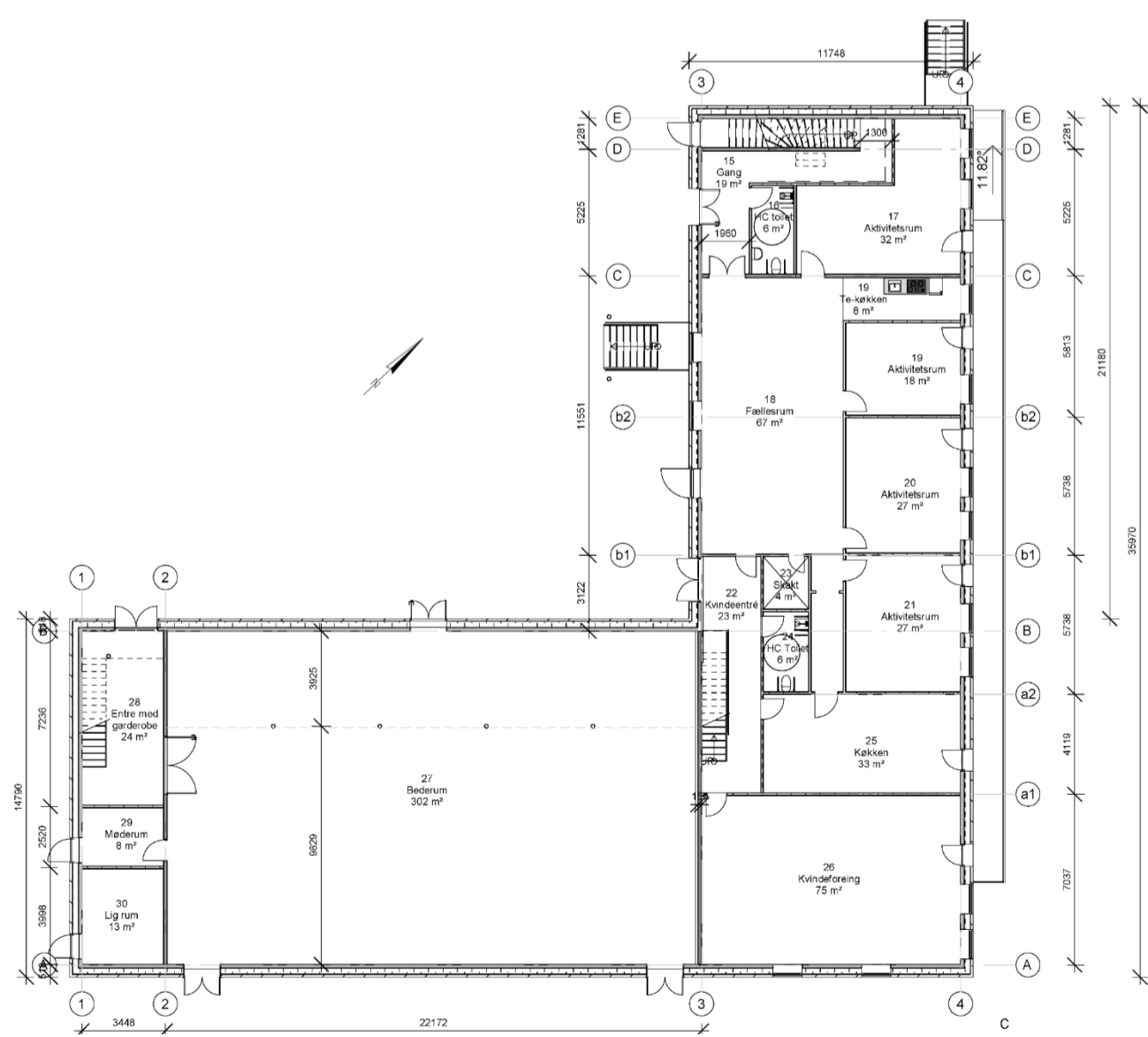
Stueplan
