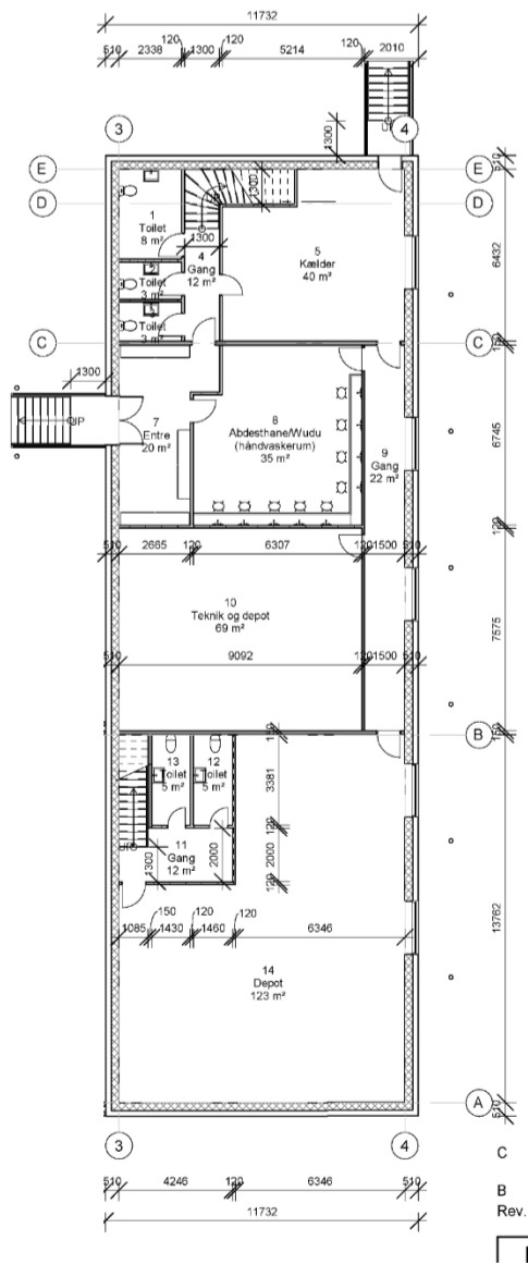
Kælderplan
