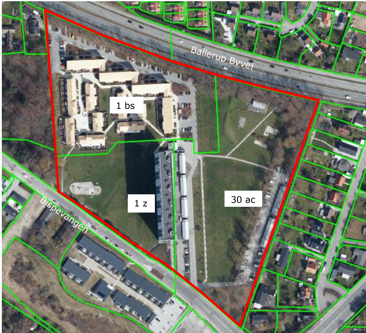
Rammeområde 3.B5 med matrikelnumre
